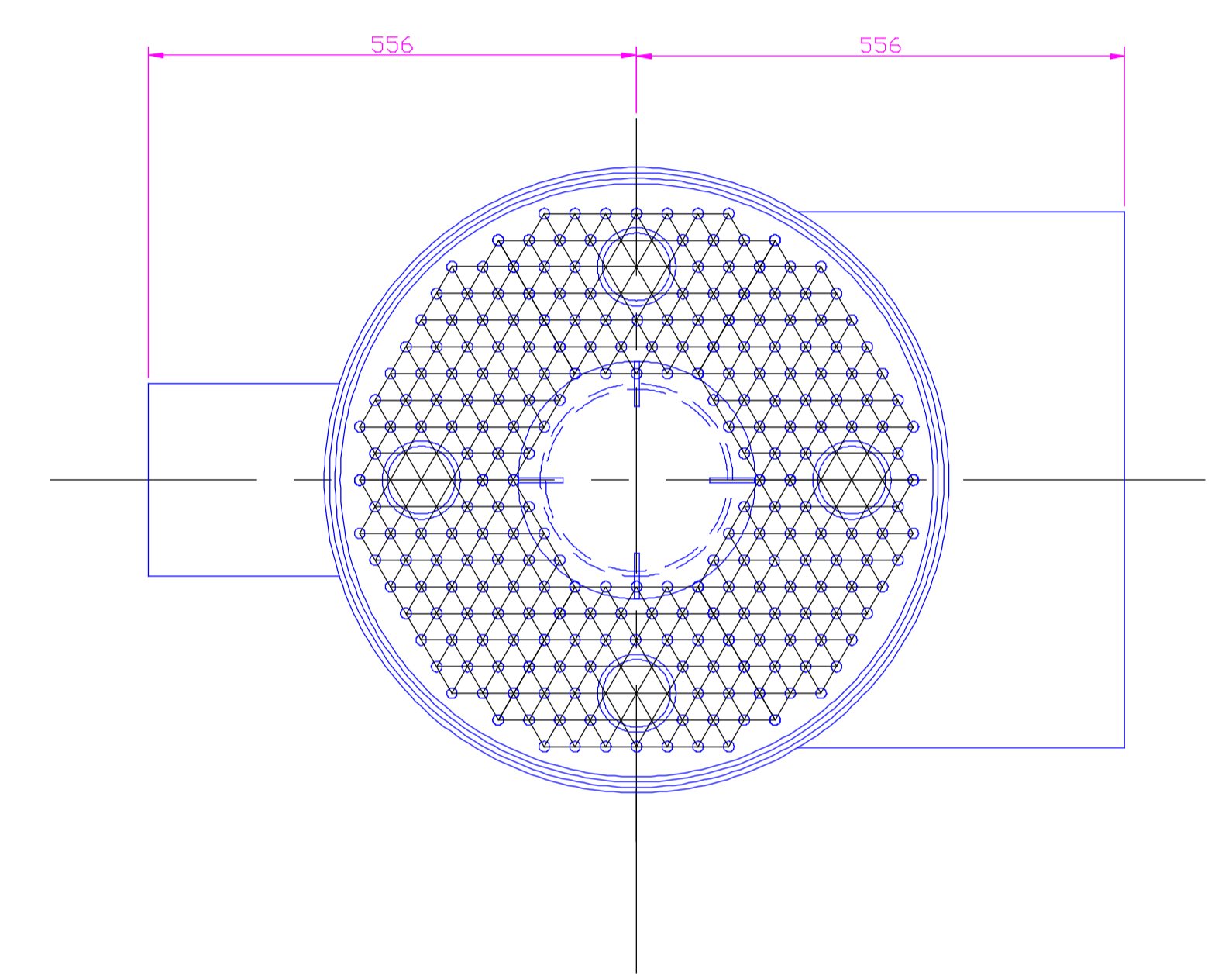
Section A-A
